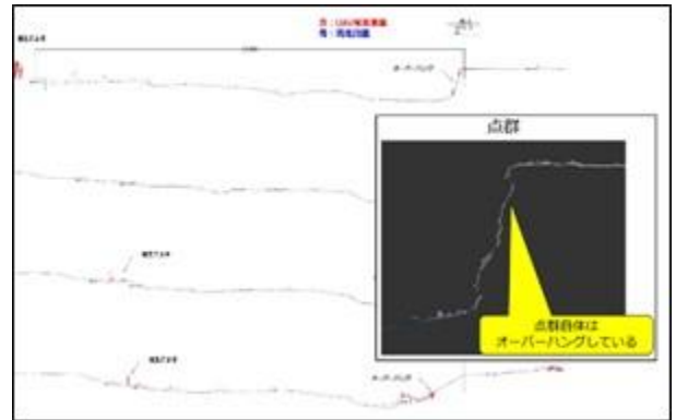
UAV 計測データからの横断面作成
